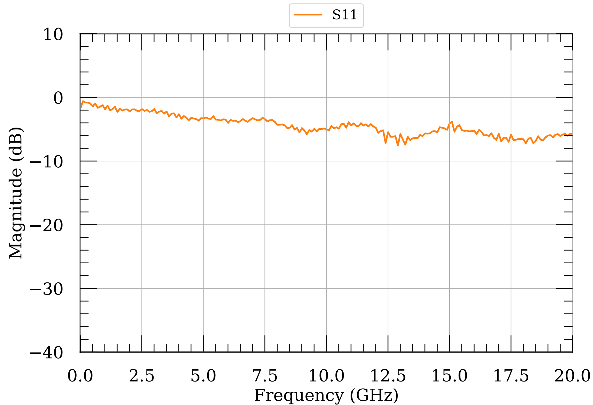
LNA S-params module068
